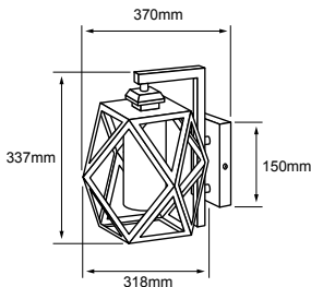
ALTER III 60FTL3434MVCA ■ Negro/Ambar POTENCIA: 60 W máx. LÁMPARA SUGERIDA: Filamento LED VOLTS: 100-240 V ~ Tipo de lámpara: Opcional (No incluida) IK: 05 Tipo de base: E27
